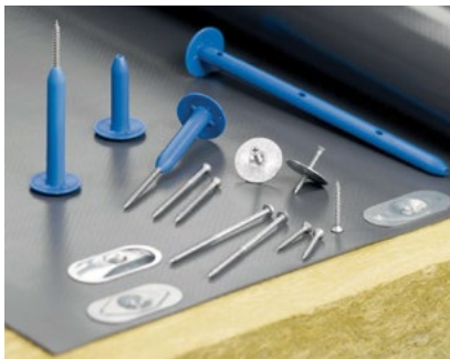
Isotak® - ekonomický systém kotvenia plochých striech pomocou skrutiek a platových teleskopov
